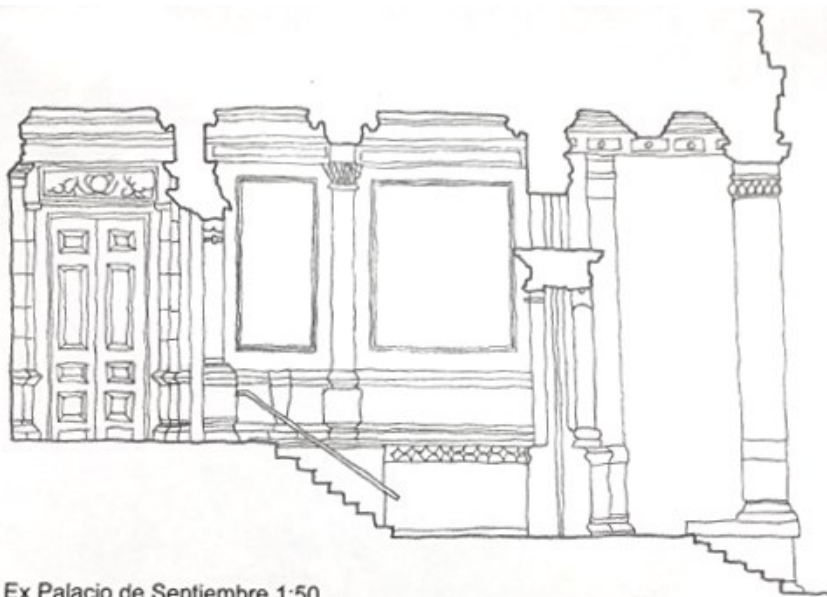
Corte Ex Palacio de Septiembre 1:50
