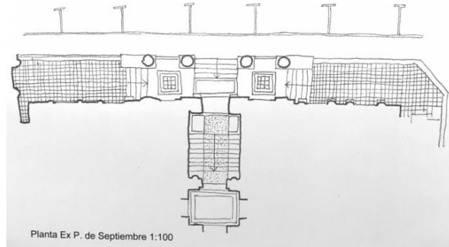
Planta Ex P. de Septiembre 1:100
