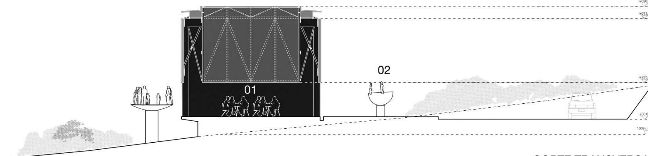
CORTE TRANSVERSAL CC' Esc. 1:100 Listado de recintos 01 Patio abierto cafetería 02 Acceso norte
